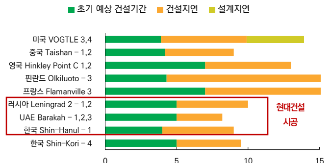
(단위: 년) 2010년 이후 글로벌 주요 지역별 원전 건설기간
